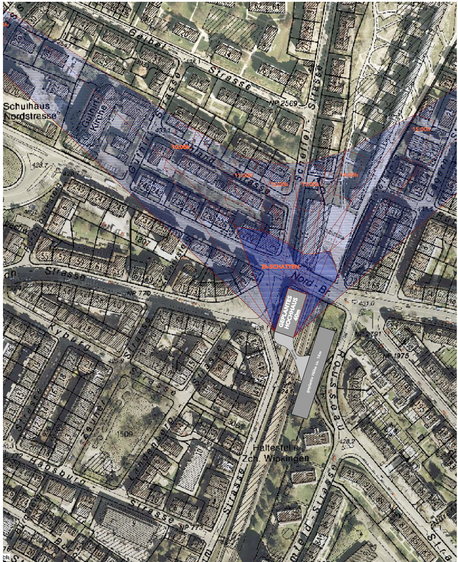
Schattendiagramm zur geplanten Überbauung des Wipkinger Bahnhofs am Rössbachplatz mittlerer Wintertag (07. Dezember)
