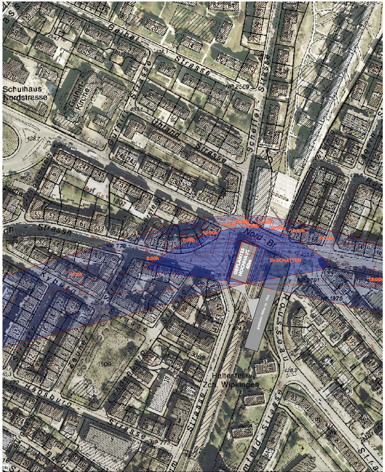
Schattendiagramm zur geplanten Überbauung des Wipkinger Bahnhofs am Röschi Bachplatz mittlerer Sommertag (30.Mai / 22.August)
